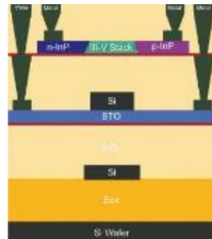
Émetteur-récepteur mono puce
